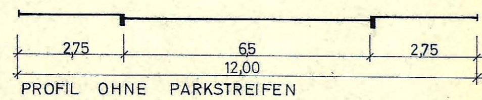
PROFIL OHNE PARKSTREIFEN
