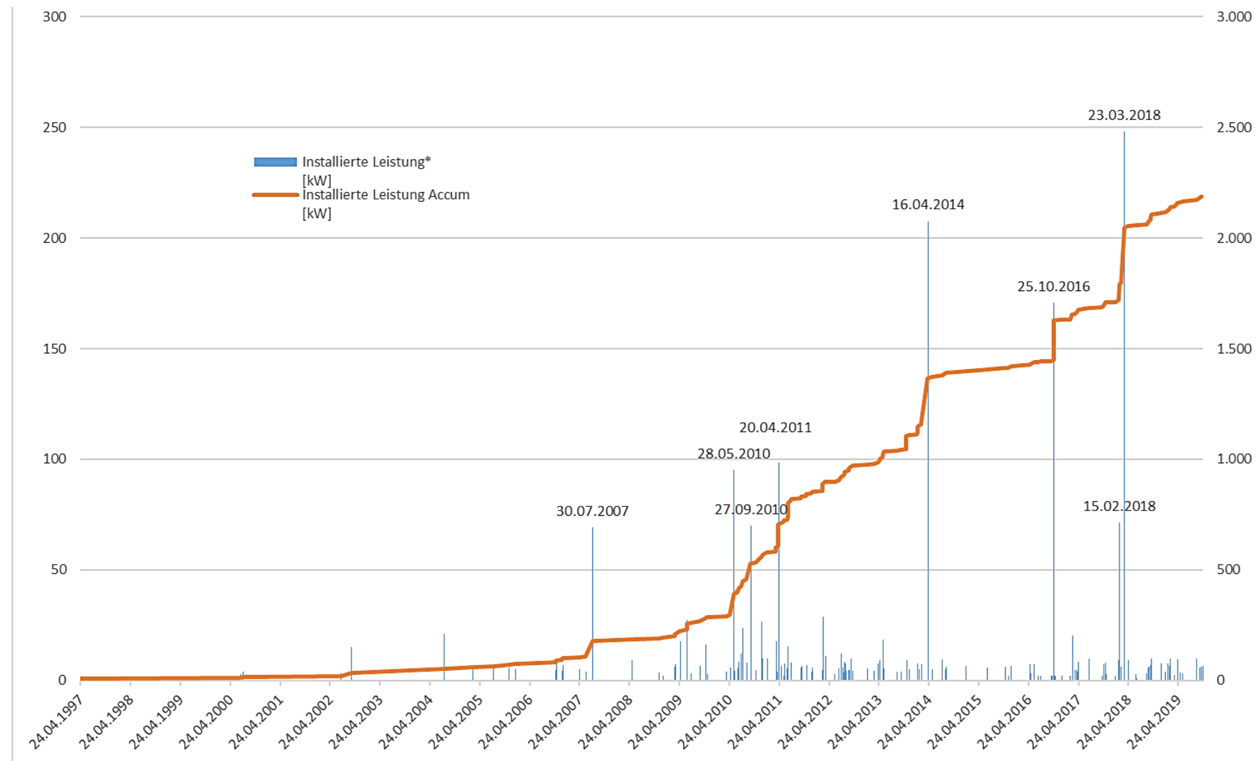
Installierte Solare Leistung [kW]
