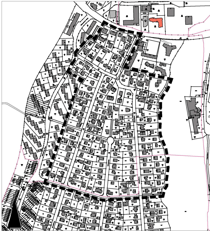
Geltungsbereich des Bebauungsplanes Nr. 110 „Hinschendorf Nord“ der Stadt Reinbek
